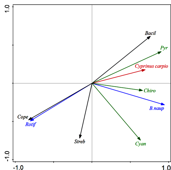
شکل ۳: نمودار دوگانه (biplot) روابط فراوانی بچه‌ماهیان کپور ( Cyprinus carpio ) و گروه‌های فیتوپلانکتونی، زئوپلانکتونی و کفزیان ( Bacillariophyta : Bacil, Cyanophyta : Cyan, Pyrrophyta : Pyr, Balanus nauplii : B.naup, Copepoda : Cope, Rotifera : Rotif, Chironomidae : Chiro, Streblosio gynobranchiata : Streb). آنالیز PCA. بردارهای مشکی، آبی و سبز به ترتیب مربوط به مواردی است که ضرایب همبستگی (پیرسون) بین ۰/۳ و ۰/۵، ۰/۵ و ۰/۷ و بیش از ۰/۷ می‌باشد.
