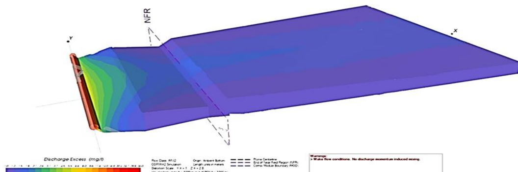
شکل ۲: مدل سه بعدی روند تغییرات غلظت نیترژن در فصل بهار
