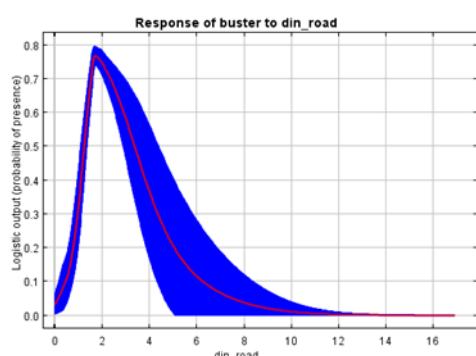
شکل ۸: بررسی نقش متغیرها در مدل‌سازی توزیع گونه‌ها (الف) متغیر ارتفاع و (ب) متغیر تراکم حمل و نقل Figure 8: Assessment of variable contributions to species distribution modeling: (a) elevation and (b) transportation network density
