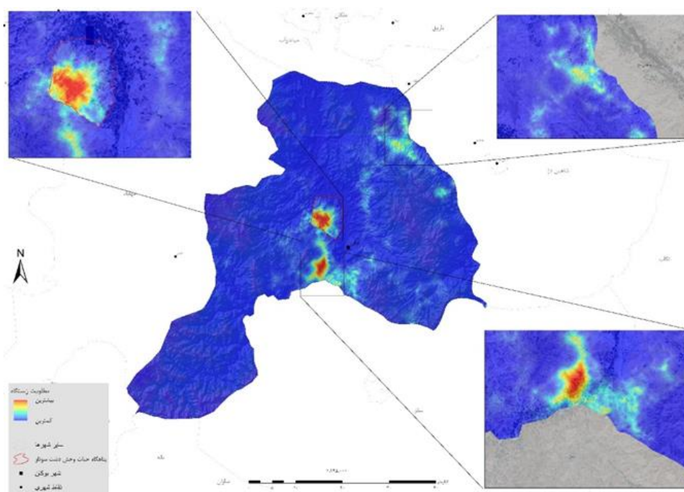
شکل ۳: موقعیت نقشه مطلوبیت زیستگاه گونه مرغ میش دشت سوتا و سایر محدوده‌های پیش‌بینی شده توس مدل حداکثر بی‌نظمی
