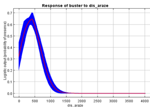
شکل ۹: بررسی نقش متغیرها در مدل‌سازی توزیع گونه (الف) متغیر فاصله از مزارع و (ب) متغیر فاصله از پناهگاه حیات وحش Figure 9: Assessment of variable contributions to species distribution modeling: (a) distance from agricultural lands and (b) distance from wildlife refuges
