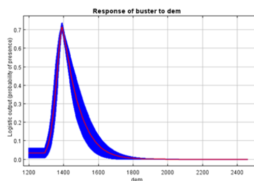
شکل ۸: بررسی نقش متغیرها در مدل‌سازی توزیع گونه‌ها (الف) متغیر ارتفاع و (ب) متغیر تراکم حمل و نقل Figure 8: Assessment of variable contributions to species distribution modeling: (a) elevation and (b) transportation network density
