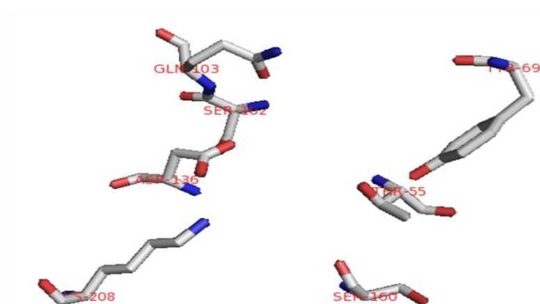
شکل ۶: محل قرارگیری و بنیان‌های تشکیل‌دهنده جایگاه فعال آنزیم ال-آسپاراژیناز B. megaterium II
