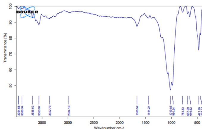
شکل ۵: طیف FT-IR نانوکامپوزیت سیپولایت/ژل رویال/نیترا نقره
