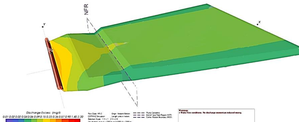
شکل ۷: مدل سه بعدی روند تغییرات غلظت فسفر در فصل پائیز
